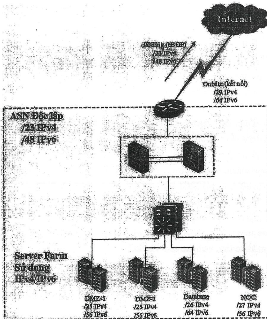
Hình 7. Quy hoạch IPv4/IPv6
