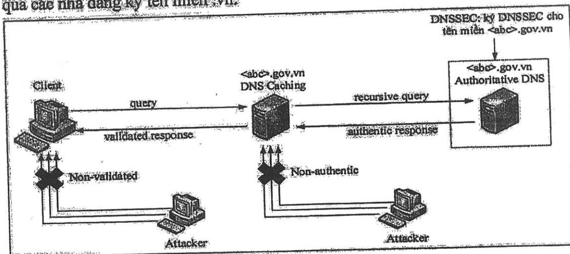
Hình 18. Triển khai DNSSEC
