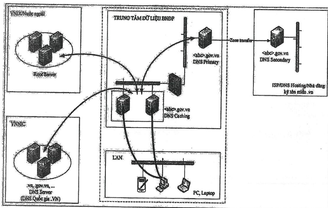
Hình 19. Mô hình tổng thể DNS Caching cho BNDP
